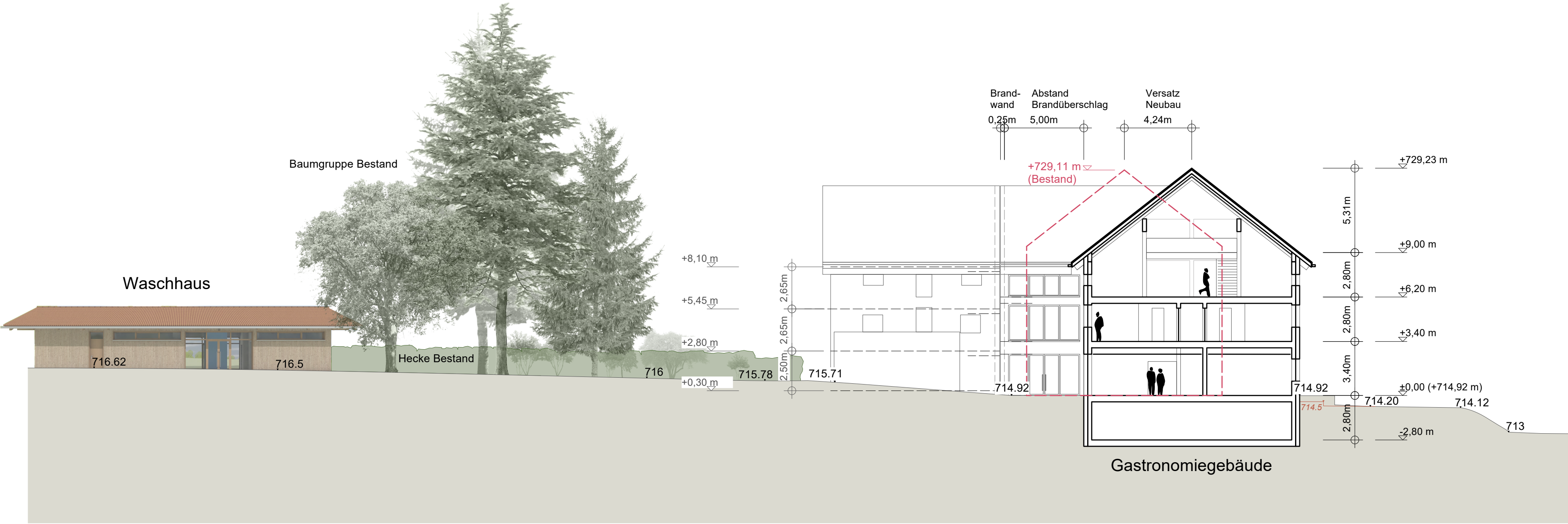
Schnitt AA' Gastronomiegebäude mit Veranstaltungsfunktion und Fremdenzimmern
