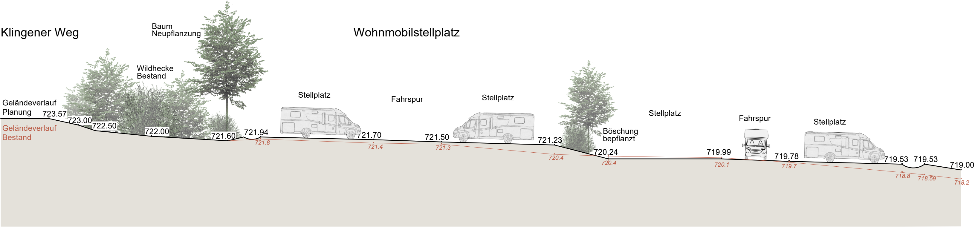
Schnitt BB' Wohnmobilstellplatz
