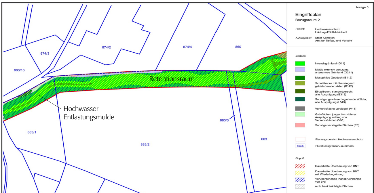
Abb. 29: Eingriffsplan Bezugsraum 2, ohne Maßstab (vgl. Anlage 5)
