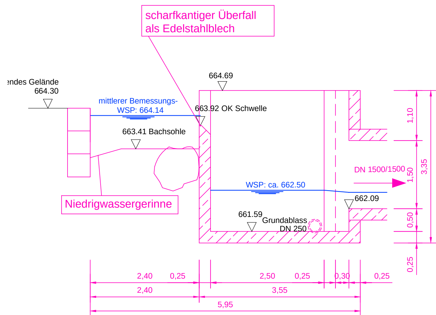
Schnitt B-B
