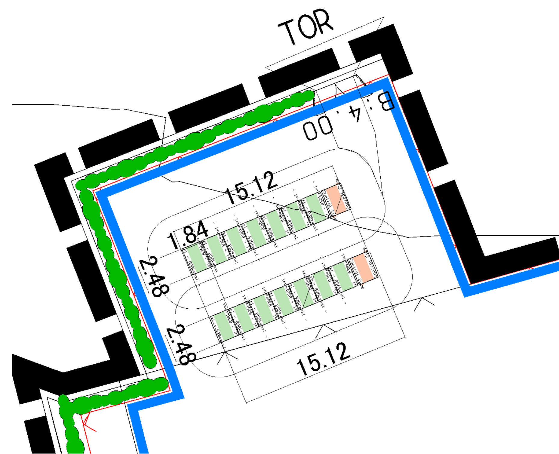
AUSSCHNITT M 1:200
