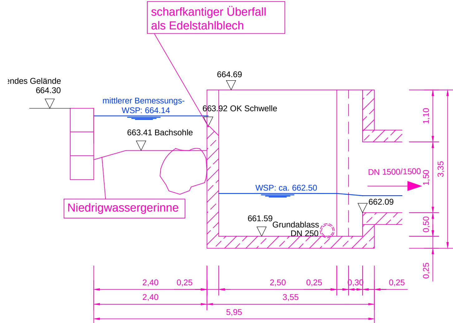
Schnitt B-B
