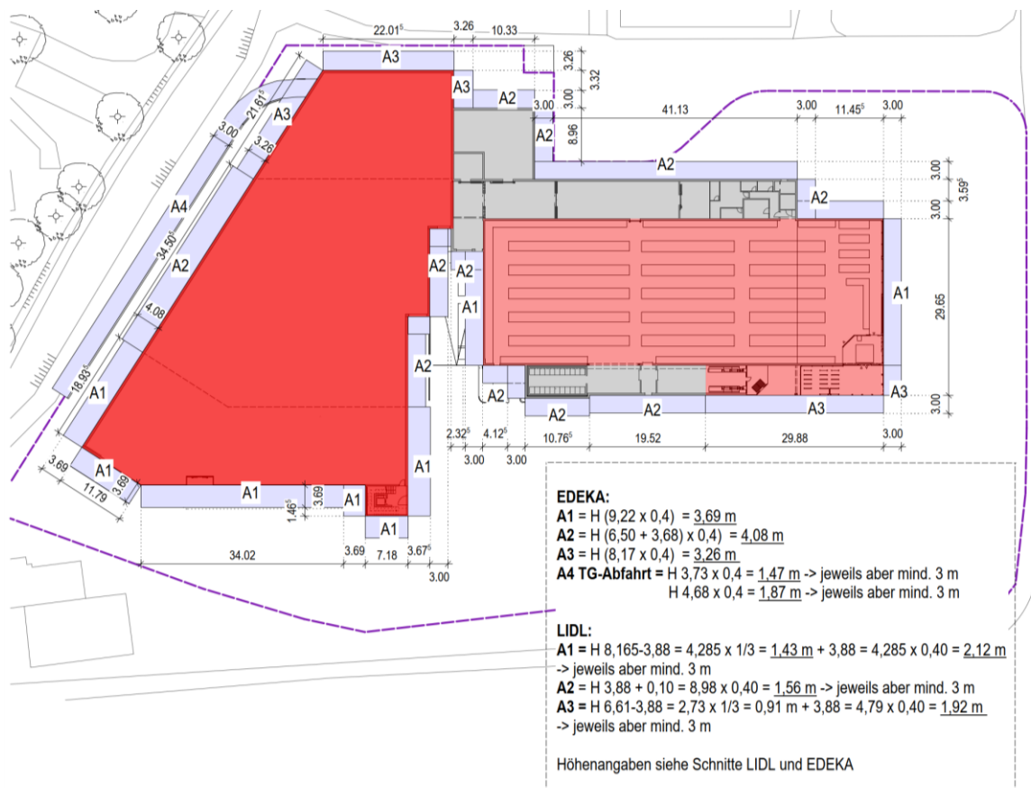
Abbildung 6: Abstandsflächenplan (Quelle: ASK Stiegeler & Klatt PartG mbH, Stand: Oktober 2024, ohne Maßstab)
