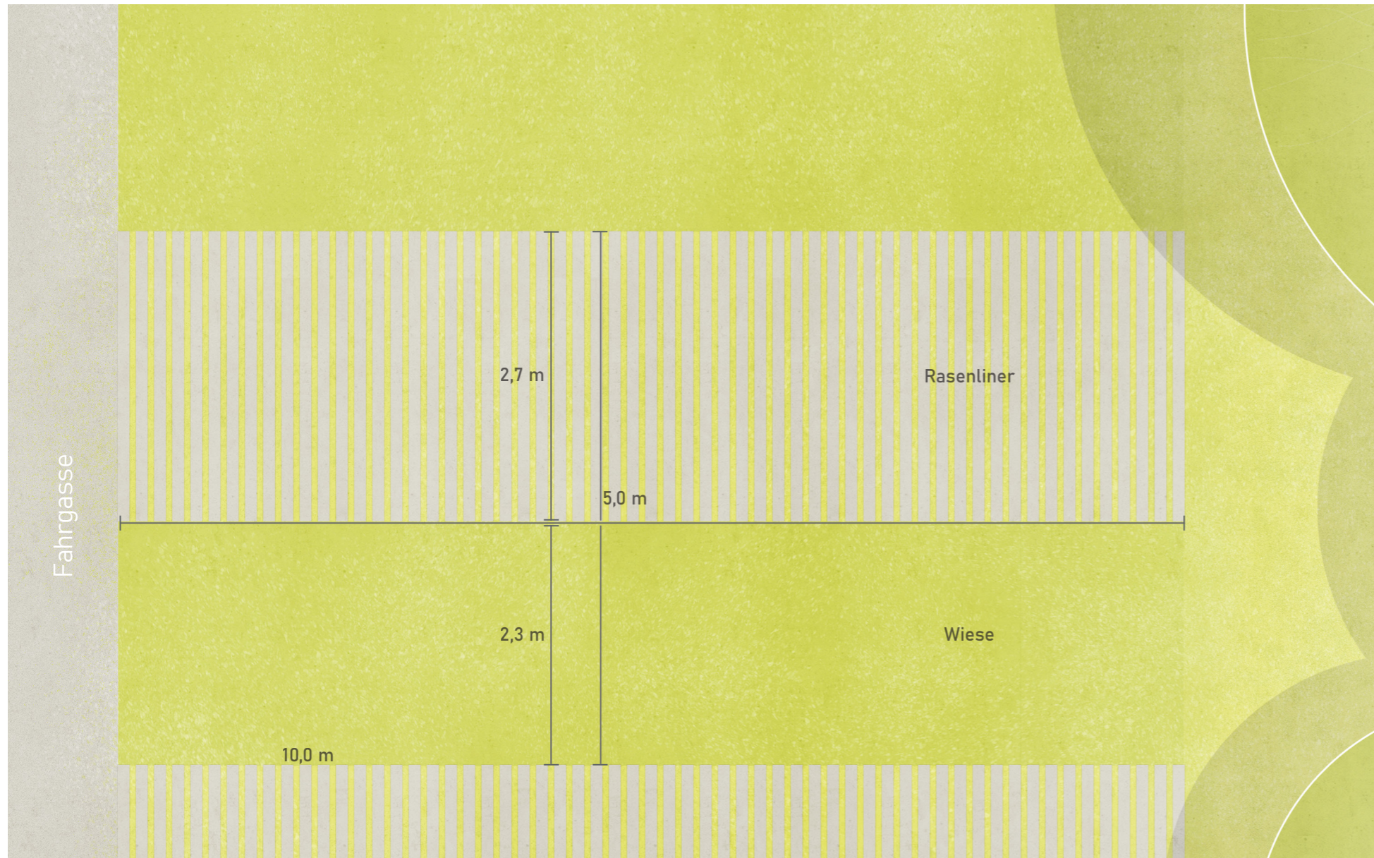
Detail Wohnmobilstellplätze M 1:50
