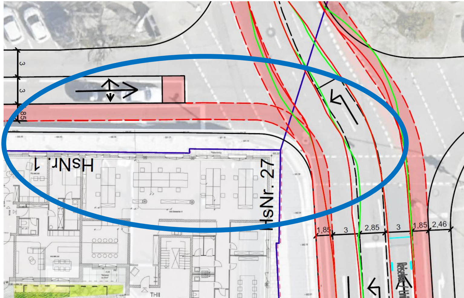
Ausschnitt Vorentwurf
