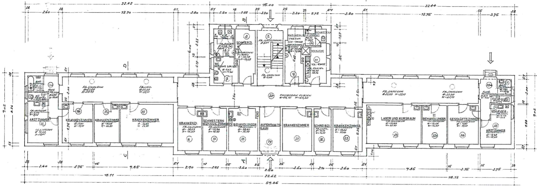
ERDGESCHOSS SÄMTL. RÄUME FÜR SAN. SCHULE
