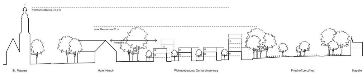
Abbildung 2: Systemschnitt (Höhendarstellung) in Nord-/Südrichtung, o.M.
