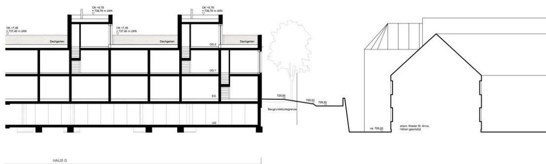
Schnitt B-B zu St. Anna
