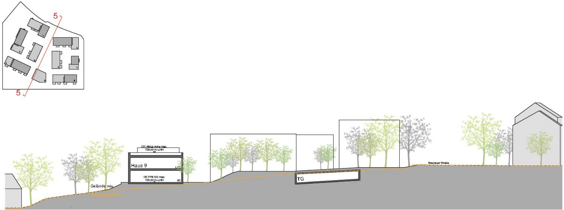
Schnitt 5-5
